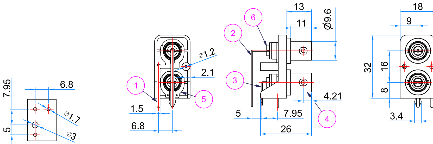
P.C.B Layout ( 1 : 1 )
