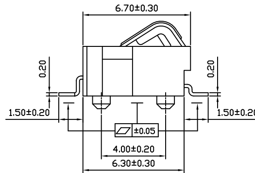
SEC: A-A
