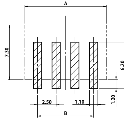
P.C.B LAYOUT
