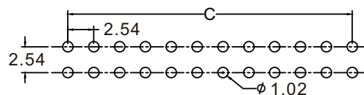
P.C.B LAYOUT
