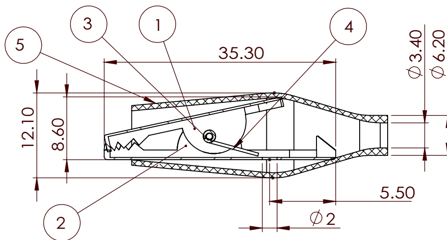
剖面圖 D-D
