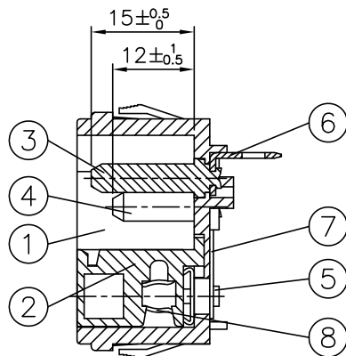
A-A 剖面
