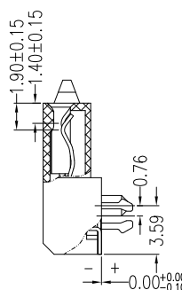
SECT A-A
