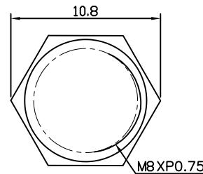
Nut
