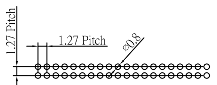
P.C.Board Layout
