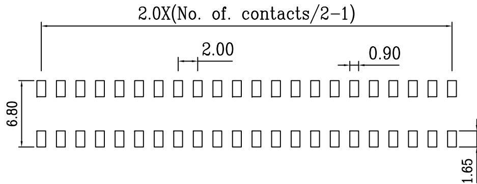
P.C.B. layout
