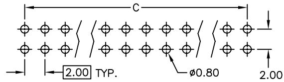
RECOMMEND P.C.B. LAYOUT
