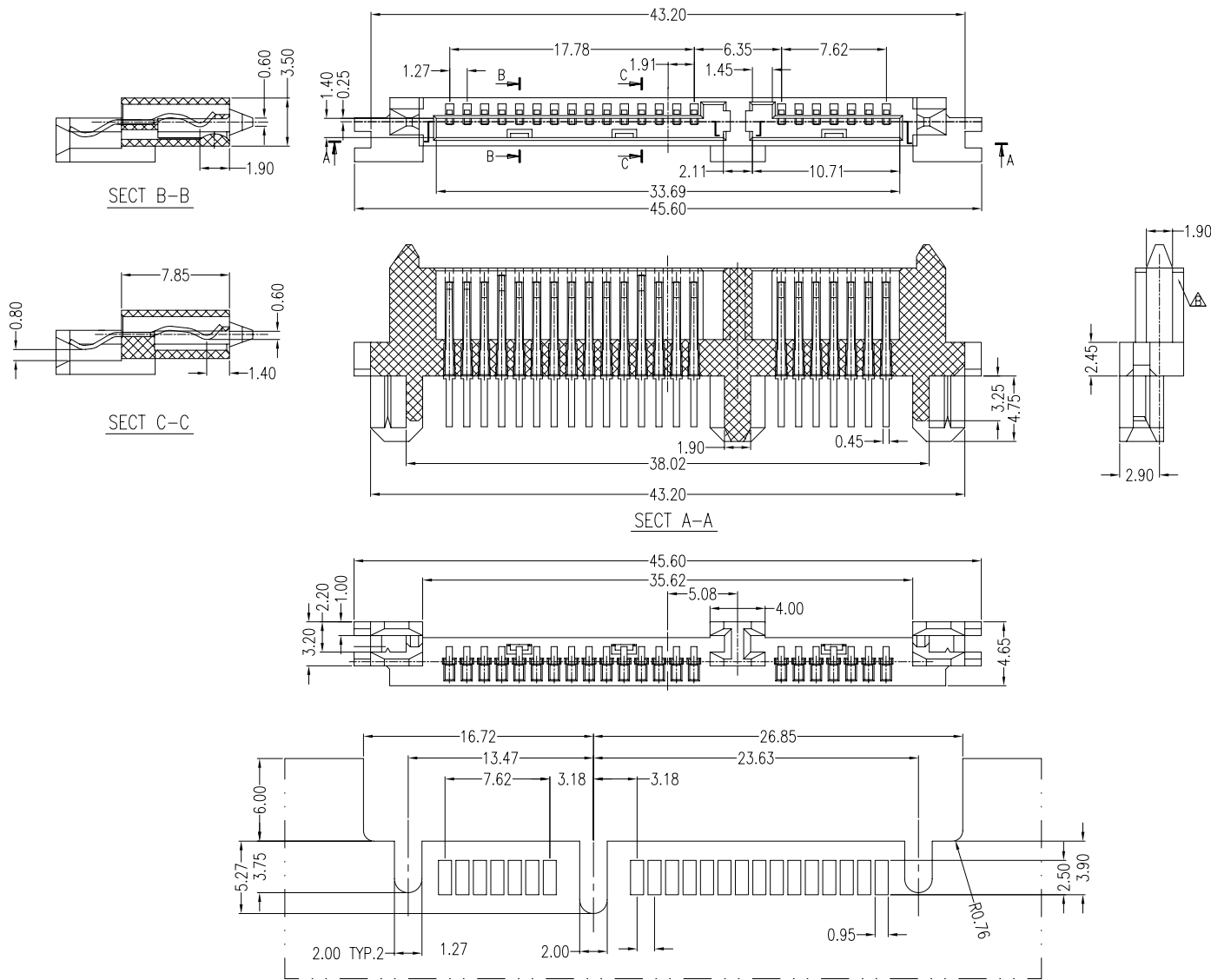
Straddle P.C.B. Layout(T=1.0mm)
