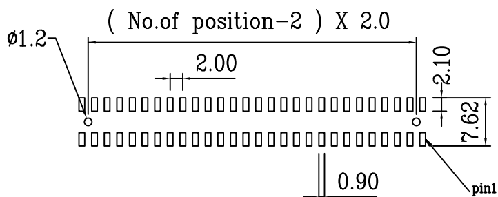
P.C.B.layout
