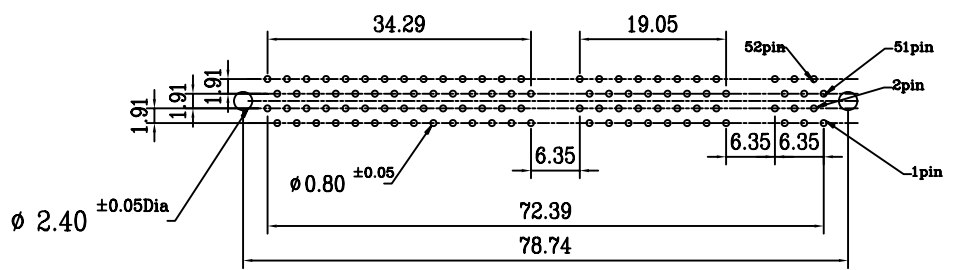
P.C.B. LAYOUT
