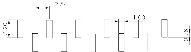
P.C.B LAYOUT
