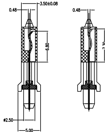
SECT A-A
