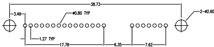
P.C.B. LAYOUT
