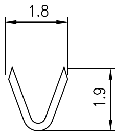
A-A SECTION
