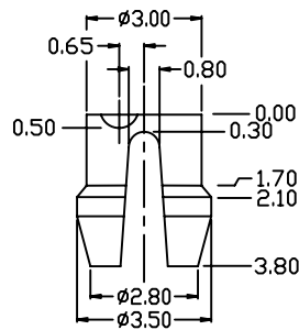
DETAIL Y
