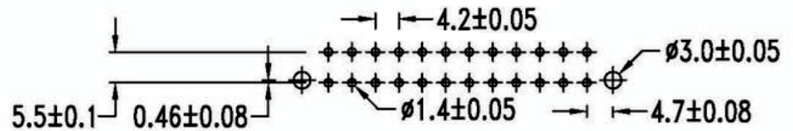
P.C.B. hole dimensions
