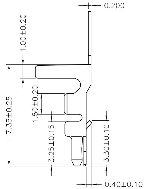
SEC:A-A
