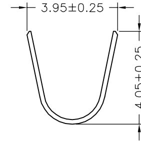
SEC:A-A
