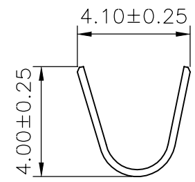
SEC:A-A
