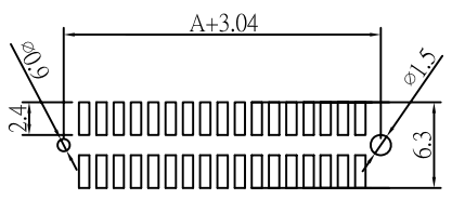
P.C.Board Layout
