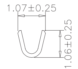
SEC:B-B
