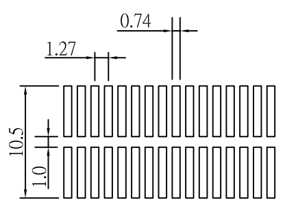
P.C.Board Layout
