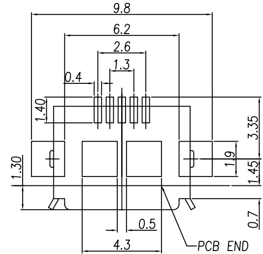
RECOMMEND P.C.B LAYOUT
