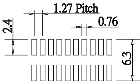
P.C.Board Layout
