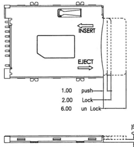
插卡示意圖
