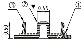
A-A section
