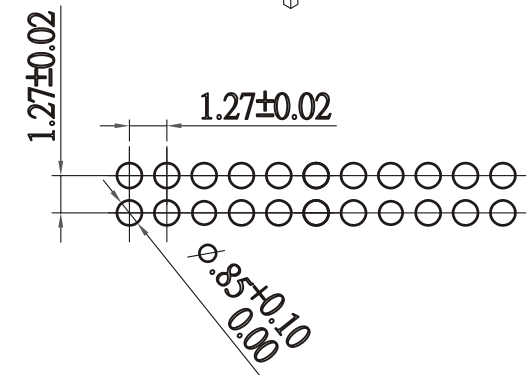
P.C.Board Layout
