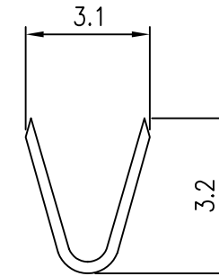
A-A SECTION
