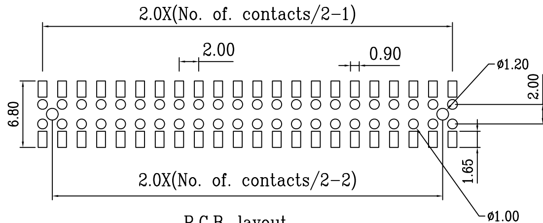
P.C.B. layout
