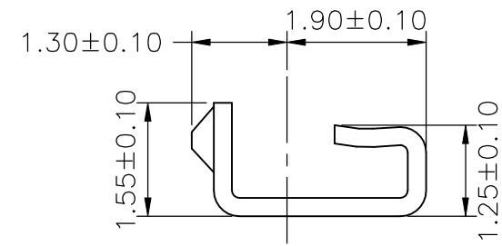
SEC:D-D
