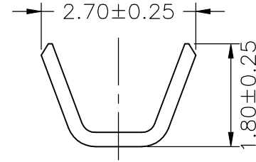
SEC:A-A
