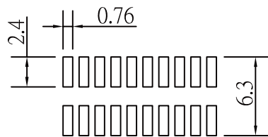
P.C.Board Layout
