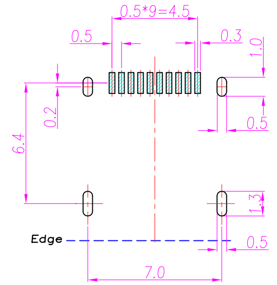
Recommend P.C.B Layout.
