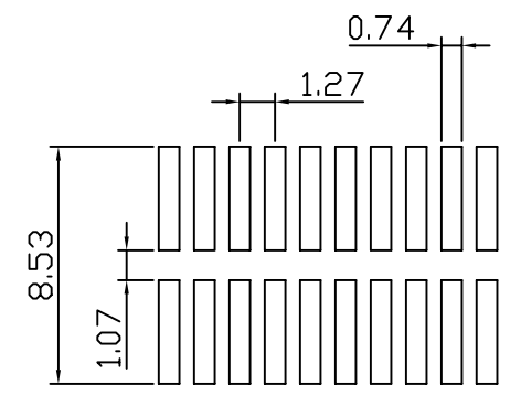
P.C.Board Layout
