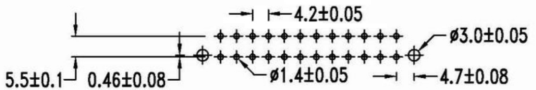
P.C.B. hole dimensions
