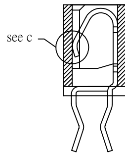
SEC A-A
