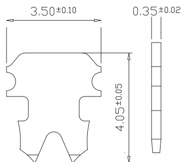
2 PRONGS FOR STRANDED WIRE 多芯線用二叉型金片
