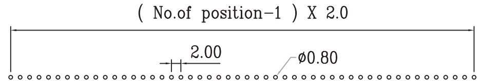
P.C.B.layout
