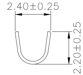
SEC:A-A
