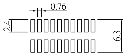
P.C.Board Layout
