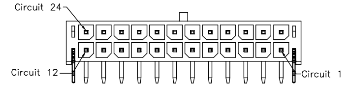
24PIN
