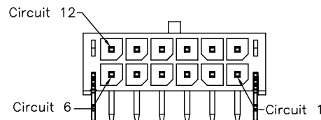
12PIN
