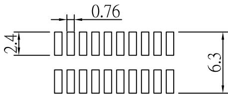
P.C.Board Layout
