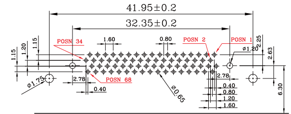
PCB EDGE
