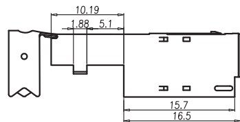
LOCK 銅管下蓋 (八件式)
