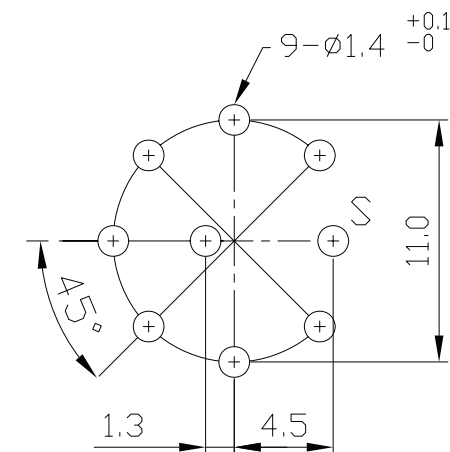
P.C.B LAYOUT(±0.1) (BOTTOM VIEW)
