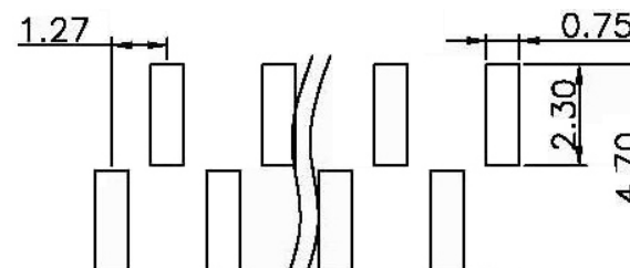
SMT TYPE P.C.B LAYOUT
