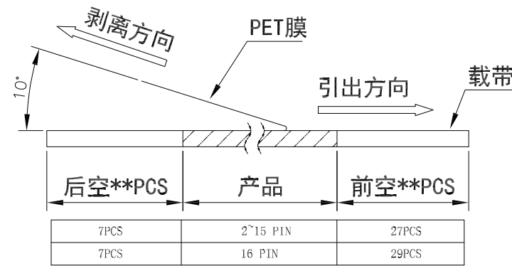
(PET膜剥离示意图)
