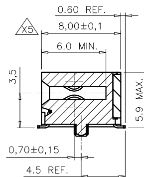
SEC. A-A
