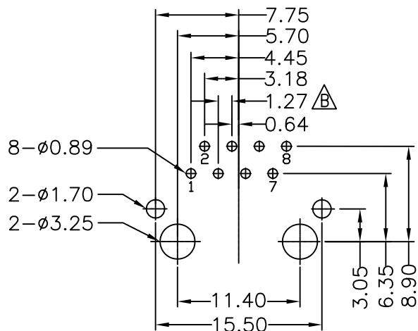
PCB Layout 2:1
